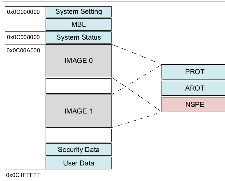
图 1-2. FLASH 规划
