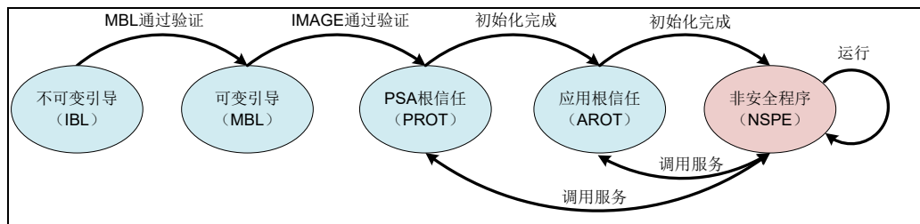
图 1-1. 引导过程
