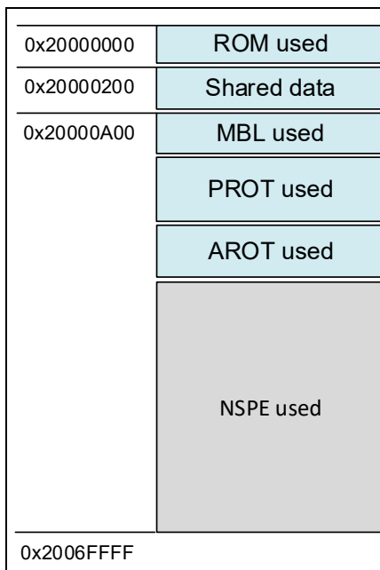
图 1-3. SRAM 规划
