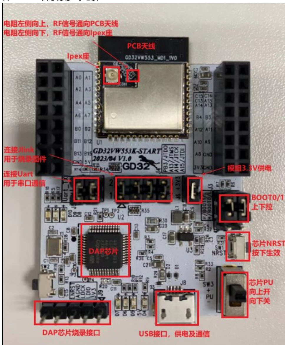
图 2-1. GD 开发板参考连接
