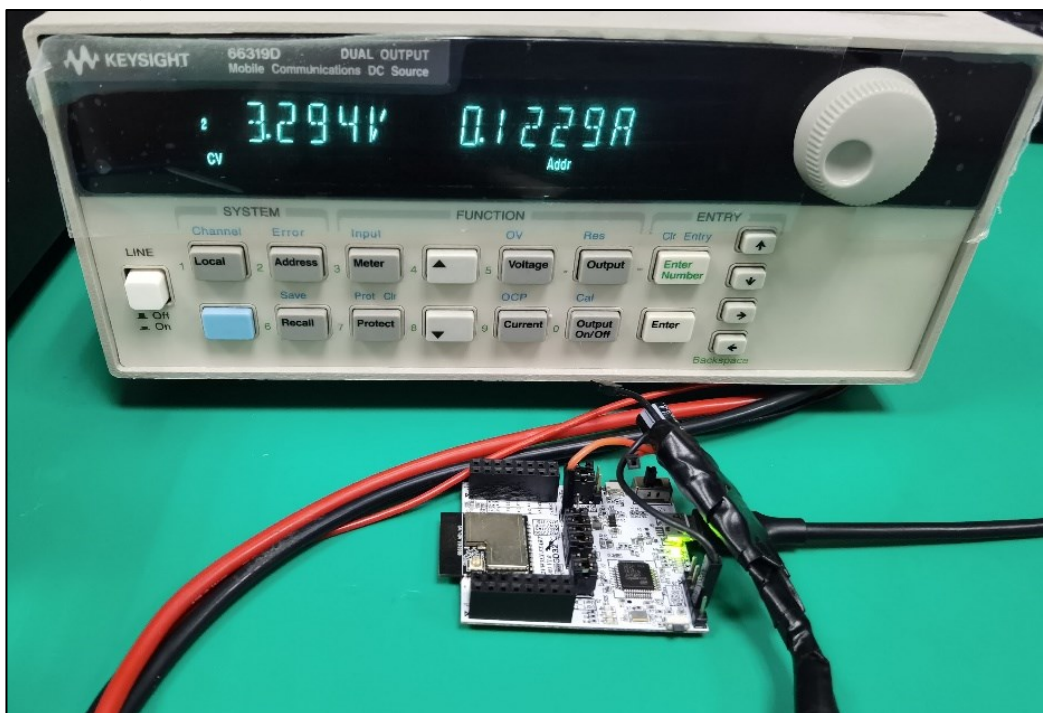
图 4-1. 功耗测试系统
