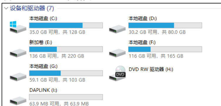
图 2-4. DAPLINK 文件夹
