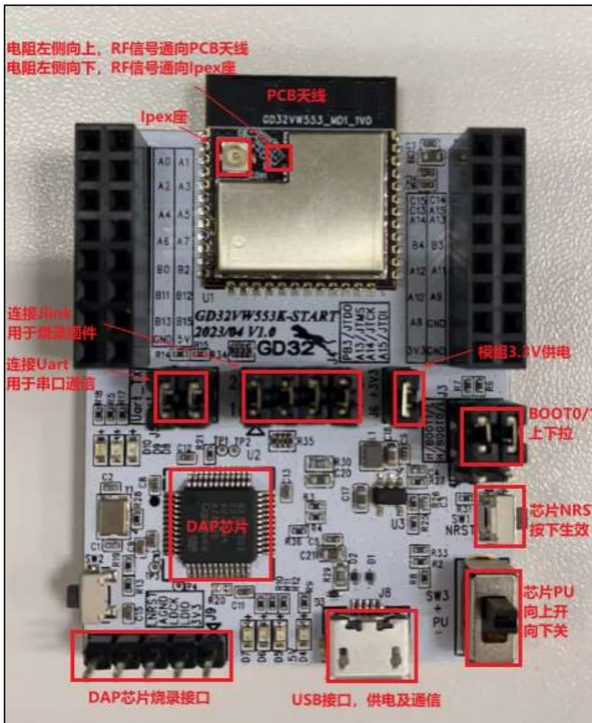
图 2-2. GD 开发板参考连接
