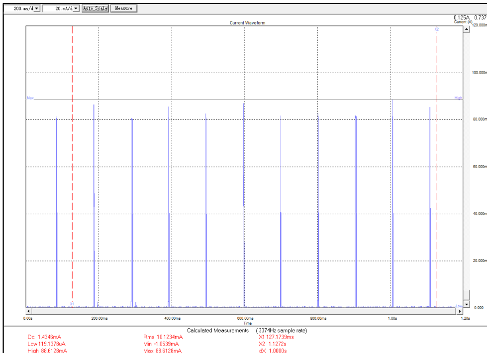
图 4-6. “DTIM=1” 功耗
